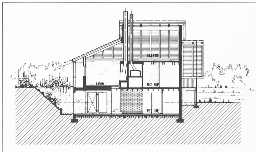
Fig. 5. — Coupe a-a.
