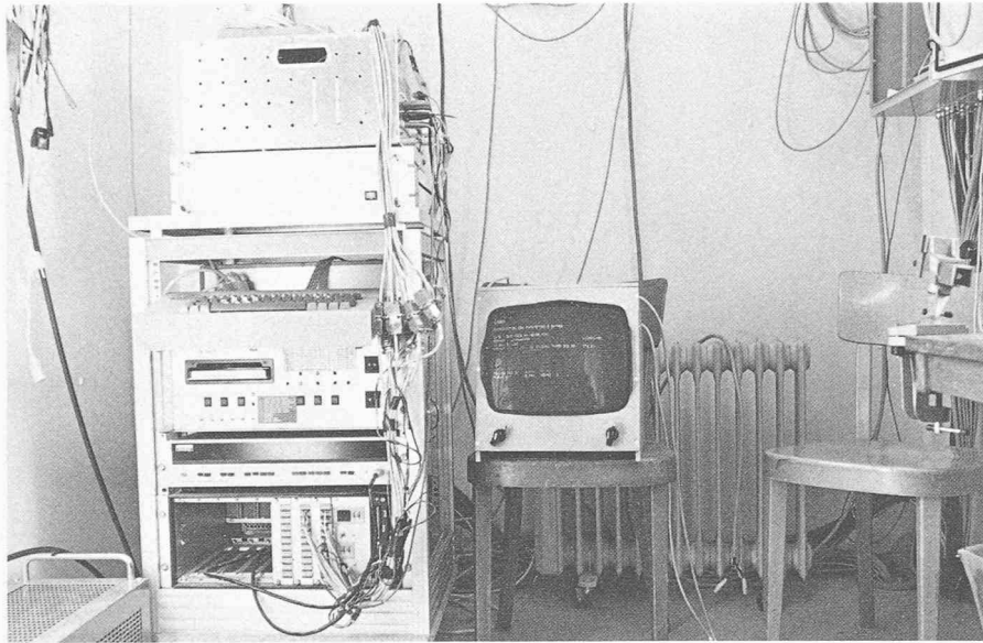
Fig. 7. — Vue intérieure de la roulotte avec l'équipement électronique du système d'acquisition de données.
