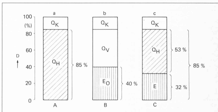
Fig. 1. — Production d'électricité avec de faibles pertes grâce au couplage énergie-chaleur. Légende : A Chaleur B Énergie électrique C Couplage énergie électrique-chaleur D Puissance calorifique du combustible
