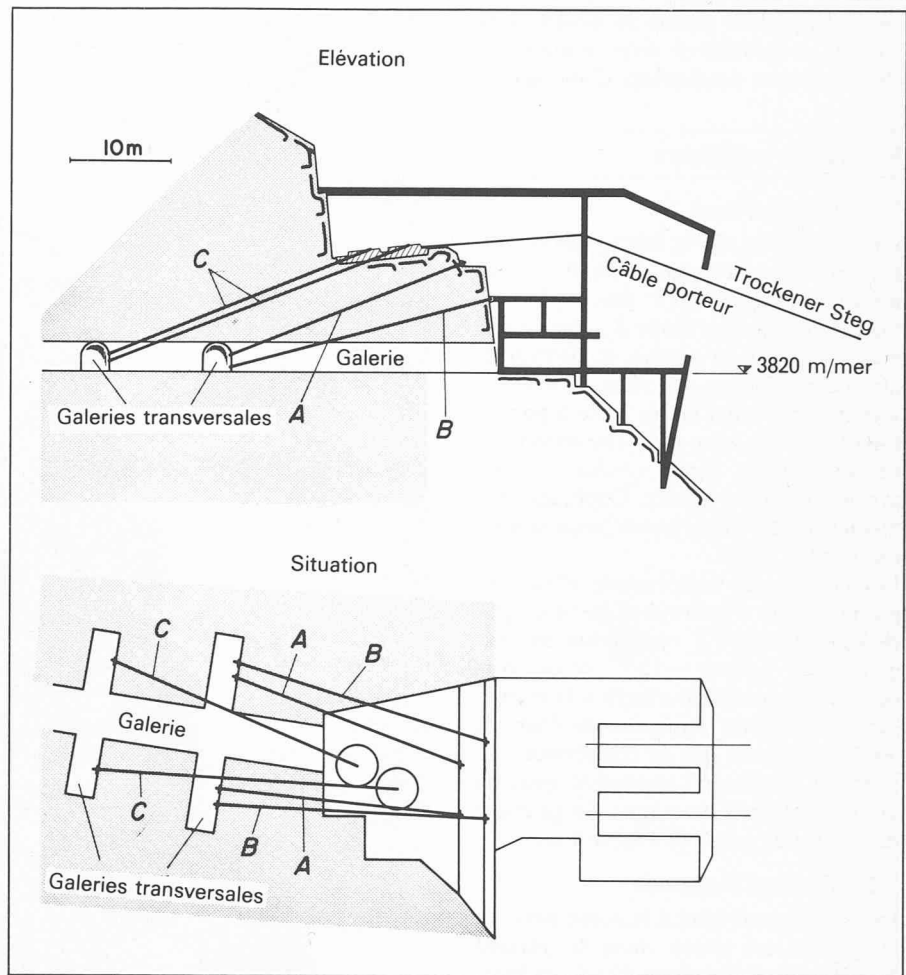
Fig. 6. — Station supérieure, ancrages (profil en long et situation).
