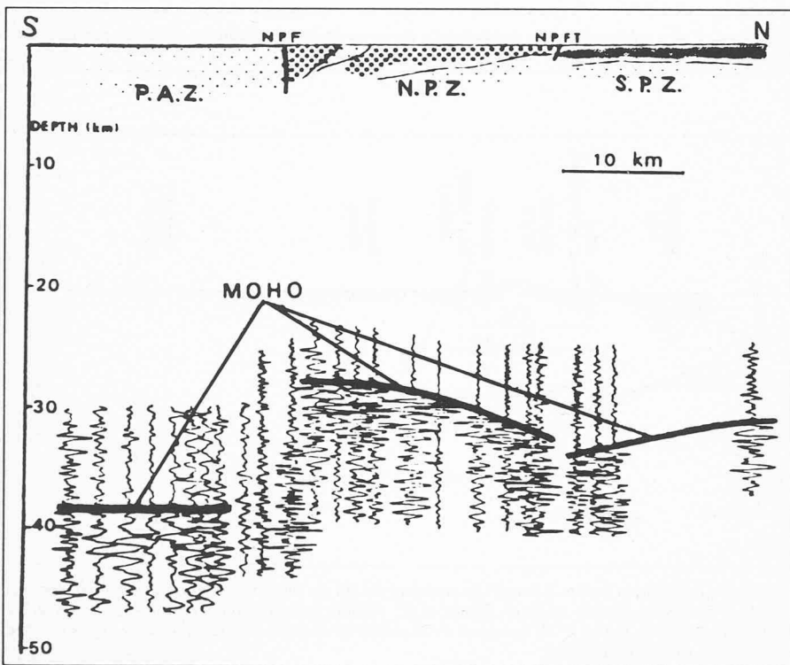
Fig. 19. — Profil de la croûte à travers les Pyrénées orientales (d'après Hirn et al., 1980). La zone de décrochement nord-pyrénéen (NPF) reflète vraisemblablement une perturbation profonde, avec un saut de la limite entre le manteau et la croûte de plus de 10 km.
