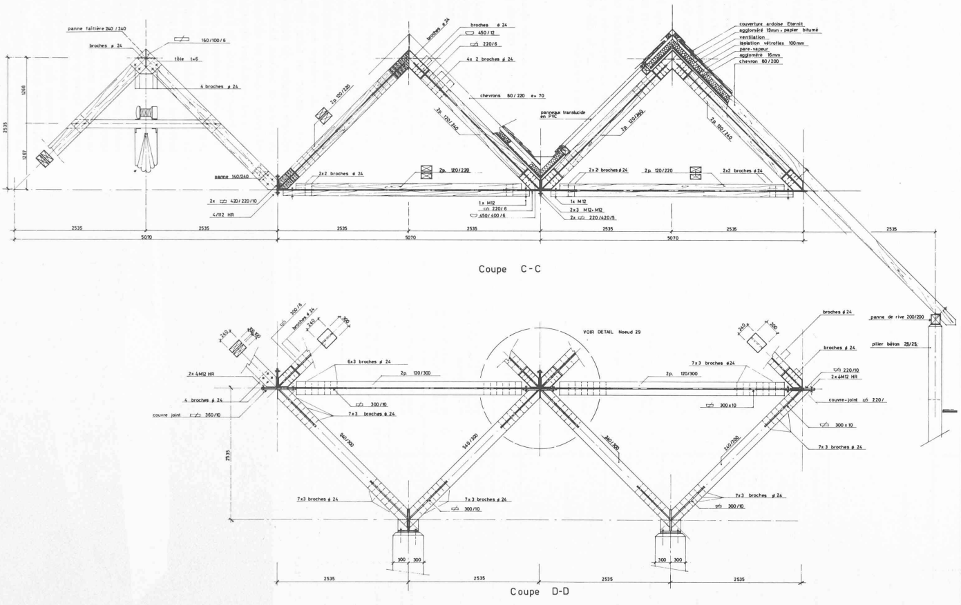
Fig. 5. — Structure secondaire supportant le niveau-dalson et coupe partielle de la structure principale.
