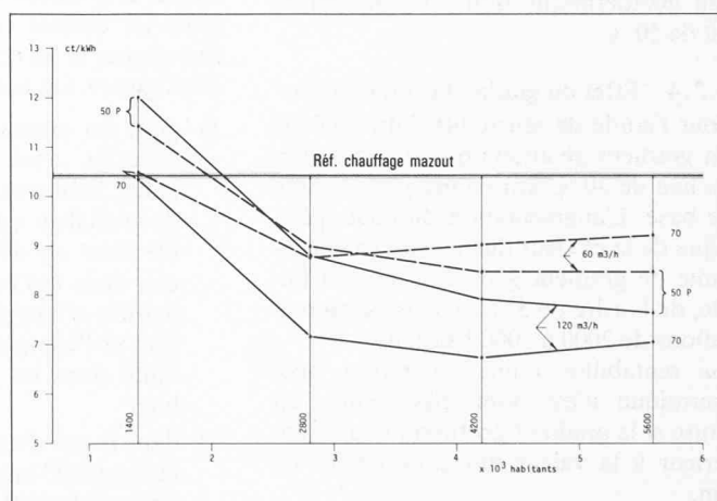
Fig. 9. — Coût spécifique de la chaleur pour une agglomération du type WE-20-A. Débit du puits: 60 m³/h (étude de base: 120 m³/h).
