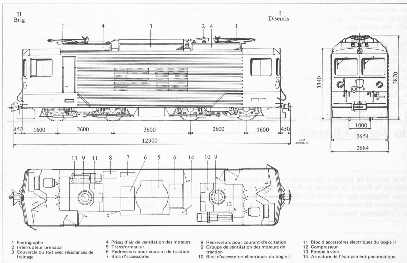
Fig. 3. — Plan-type des locomotives Ge 4/4 III n°s 81 et 82.
