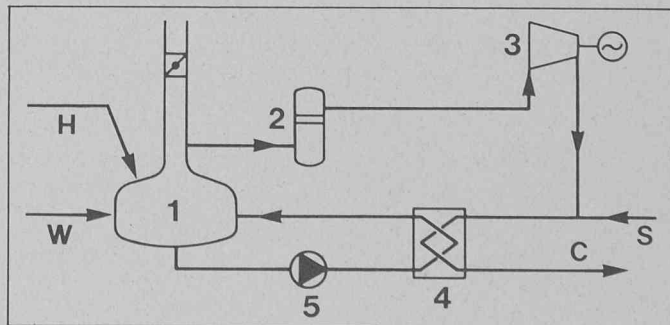
Récupération de chaleur dans les brasseries par recompression des buées.
