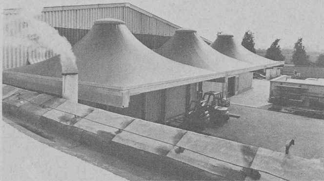
Toiture expérimentale en tissu, à Krefeld (RFA).
