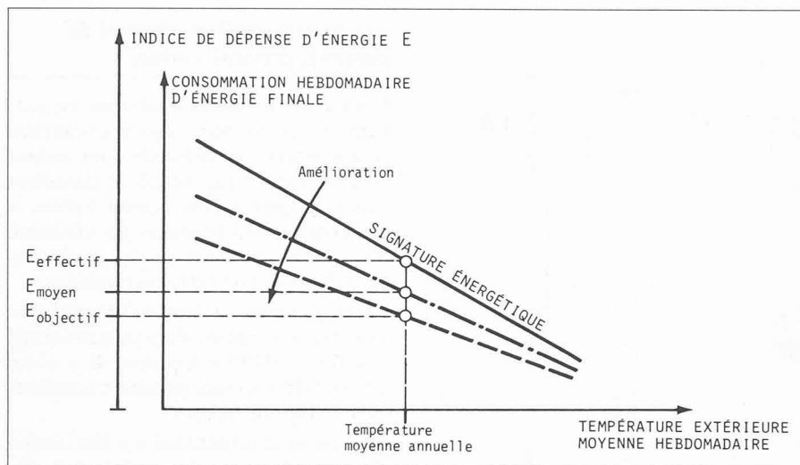
Principe du relevé de consommation hebdomadaire.
