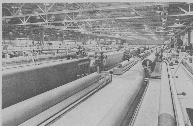
Installation de machines à tisser Sulzer de l'Amoco Fabrics à Gronau (D).
