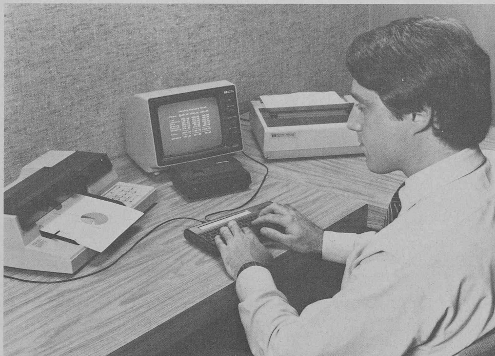
Grâce à l'interface HP-IL, le nouvel ordinateur portable à batteries HP-75C (au centre) peut commander des périphériques fort divers, tels que table traçante, écran, unité de cassettes, etc.
