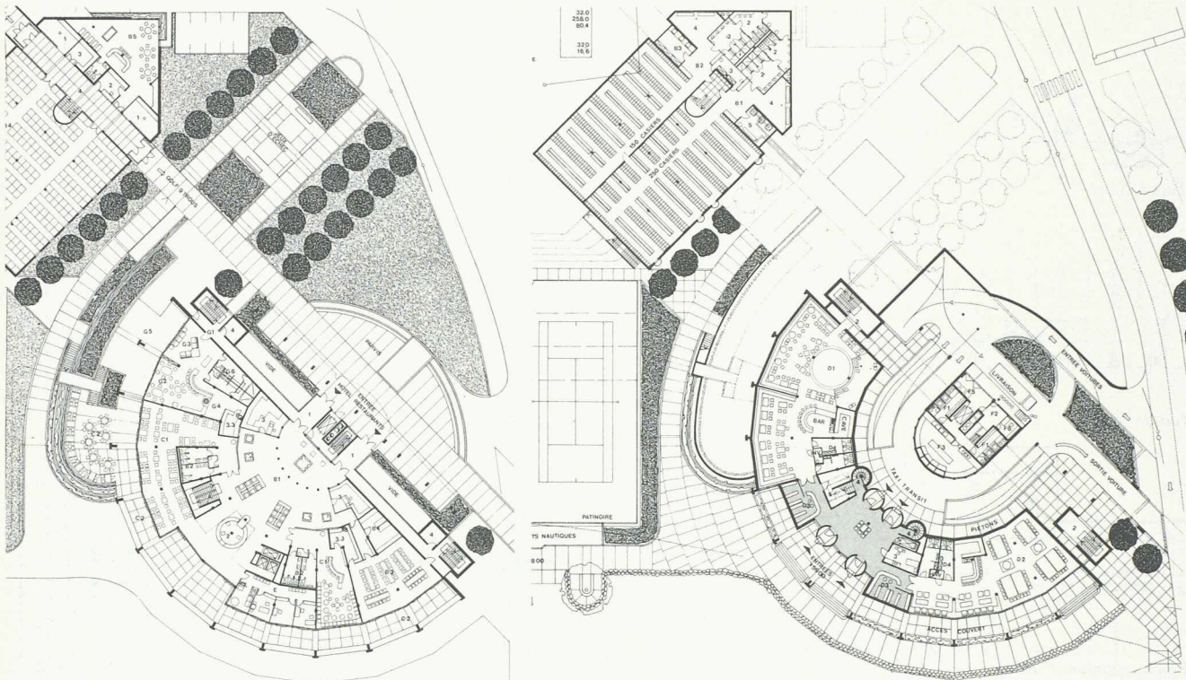
Rez-de-chaussée supérieur 1: 1000
