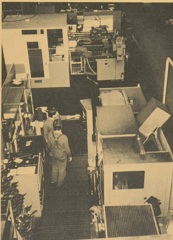
«Ilôt de fabrication autonome» équipé de machines d'usinage. Au fond, à gauche, la cabine de commande connectée à l'ordinateur pour la programmation et l'ordonnancement des ordres.
