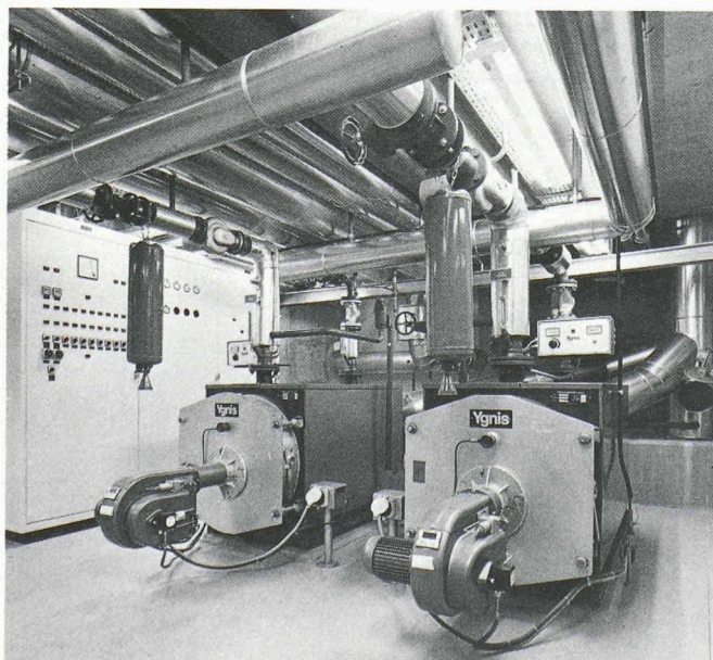
Fig. 11. — La chaufferie : seulement deux chaudières de villas... Consommation : environ 15 000 litres par an pour plus de 50 000 m 3 .
