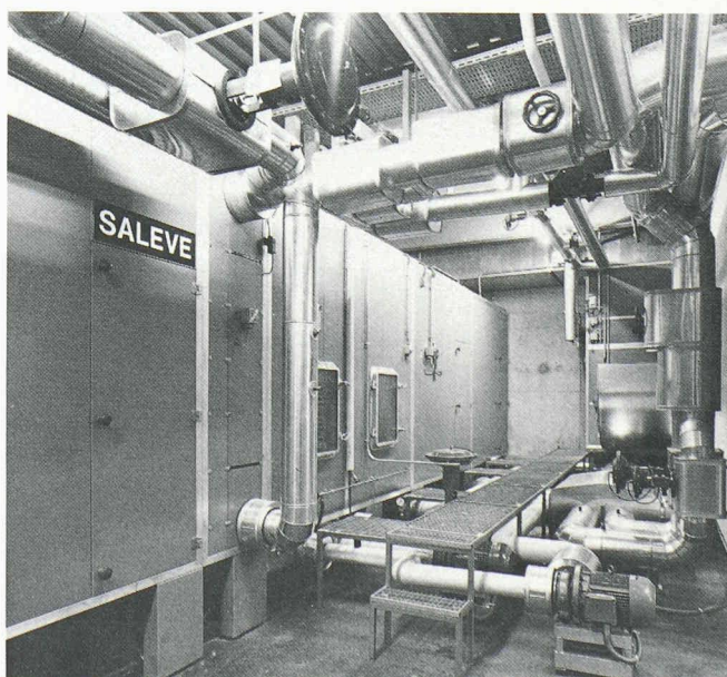
Fig. 12. — Centrale de ventilation : l'un des deux monoblocs de traitement de l'air primaire.
