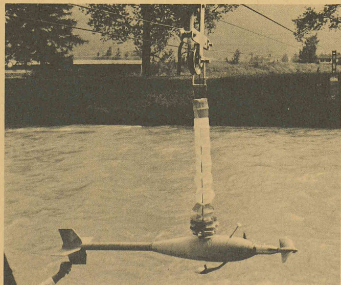
Le moulinet, fixé sur la partie droite du saumon, tourne à une vitesse qui est fonction de la vitesse de l'eau. Le saumon, muni d'ailerettes stabilisatrices, permet d'immerger et de stabiliser le moulinet dans le cours d'eau à l'endroit désiré. Les impulsions produites par le moulinet et le détecteur de fond (visible sous le saumon) sont transmises en surface par un câble électrique.
