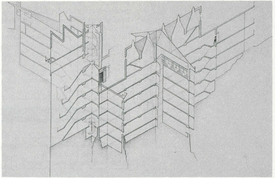
Coupe axonométrique.
