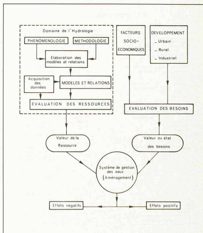
Fig. 2. — Place de l'hydrologie dans l'aménagement des eaux.
