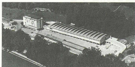
3102 Bern 2, Engehalde 1948–50 PTT-Engelhalde, Bürotrakt und «Ochsenaug-Shedhalle», Arch.gem. Daxelhofer H., Hostettler H., Indermühle P., Ing. Steiner & Stähelin
