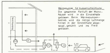
2113 Ittigen 1981-82 Wärmepumpen für bivalenten Betrieb, Mehrfamilienhäuser, Ittigenstrasse 12, 12a, Niesenweg, Ing. Kurz Markus
