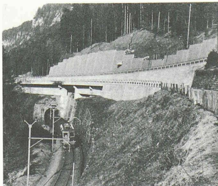
0121 Därli 1967-72 Autobahn-Stützmauern, Anschluss Ost, Stämpfli AG und Staudacher & Siegenthaler
