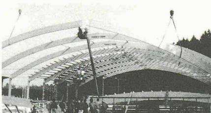
9119 Langenthal 1982-84 Überdachung Kunsteisbahn, Ing. Duppen-thaler + Wälchli
