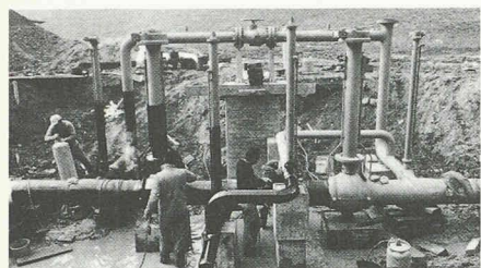
3190 Bern 6, Riedern 1980 Gasdruck-Reduzierstation, Reduktion von max. 70 bar auf max. 25 bar, Ing.-gem. Emch & Berger, Suselectra
