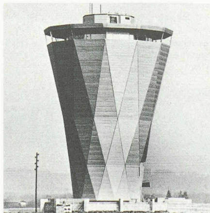
4070 Gimmiz-Walpertschwil 1970–74 Hochreservoir Gimmiz, einziges bernisches Hochreservoir La seule tour d'eau du canton; Ing. Ryser AG, Arch. Gaudy Gianpeter
