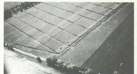
4092 (Seeland) Ins 1978–85 Detailentwässerung, kombinierte Drainage Sammler/Schlitzdrain mittels Drainfräse Hoes Gigant, Ing. Guggen + Lüscher (Mitarbeit Gemeindeingenieure Ins und Gampele sowie J.P. Zmoos)
