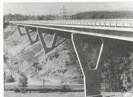
2122 Worblaufen 1960-61 N1 grosse Autobahnbrücke Worblental, Ing. Kipfer Paul (Mitarbeit Wanzlerried), Publ. Strasse und Verkehr 12/1961
