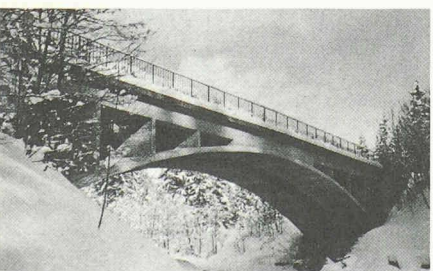
0190 Adelboden 1930 Spitalbrücke, 3 km unterhalb Adelboden (Kantonsstrasse), Ing. Maillart Robert, Publ. Bauzeitung April 1938
