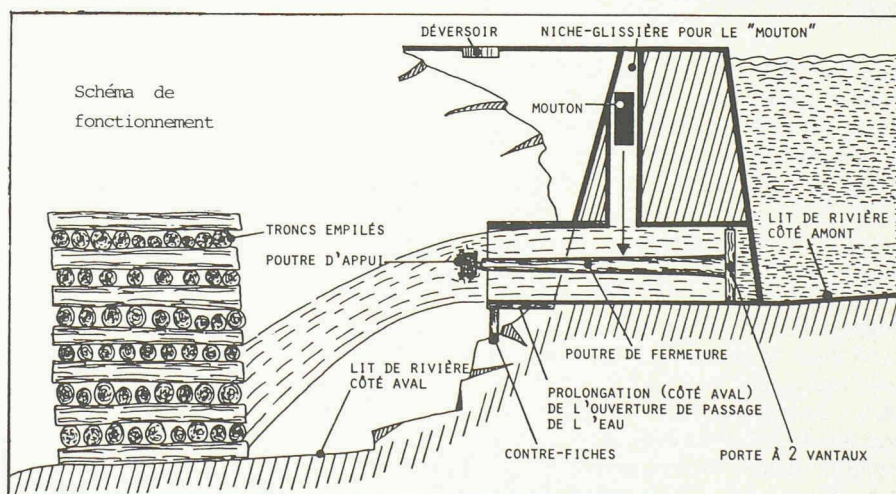
Schéma de fonctionnement du barrage.
