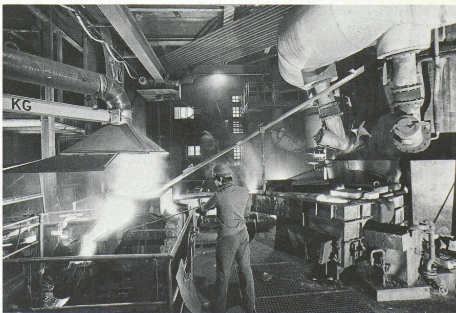
La capacité de fusion du nouveau cubilot de Choindenz atteint 28 tonnes à l'heure. L'installation permet une exploitation plus économique du fait que le coke est utilisé intégralement pour l'énergie de fusion, que les gaz servent à chauffer le four à recuire (substitution du pétrole) et qu'il est employé une technique efficace de commande et de réglage. La protection de l'environnement a fait l'objet d'une attention particulière : les émissions de poussières ont pu être réduites de 90 %, celles de monoxyde de carbone et d'anhydride sulfureux de 95 %.
