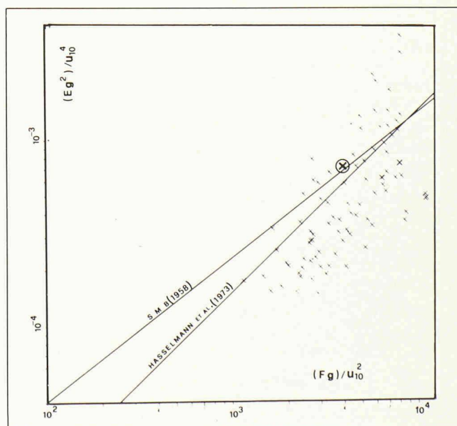
Fig. 5. Evolution de l'énergie totale E , des vagues en fonction du fetch F , et de la vitesse du vent u_{10} , sous la forme adimensionnelle, pour les données enregistrées à Buchillon. Elles sont comparées avec la relation de Hasselmann et al. (1973) et celle de SMB (1958). Le symbole (x) correspond au spectre d'énergie présenté dans la figure 3.
