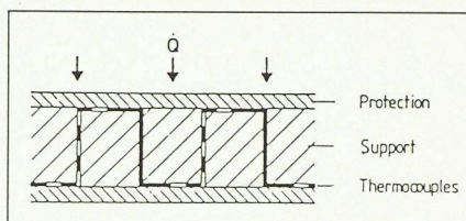
Fig. 2. — Schéma de principe de flux-mètres.
