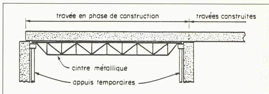
Fig. 4. — Construction travée par travée sur cintre autoporteur.
