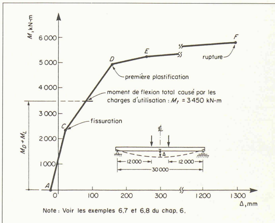
Fig. 6. — Courbe M - calculée.
