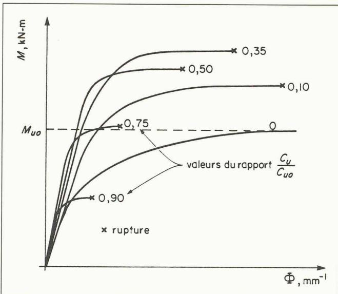
Fig. 13. — Relations moment-courbure d'une section travaillant en compression-flexion.
