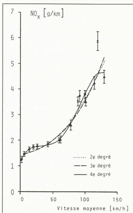
Fig. 2. — Influence de la vitesse moyenne sur les coefficients d'émission d'oxydes d'azote des voitures de tourisme (régressions polynomiales des 2 e , 3 e et 4 e degrés).
