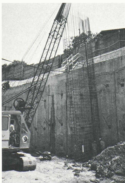
Fig. 6 et 7. — Paroi à contreforts côté amont.
