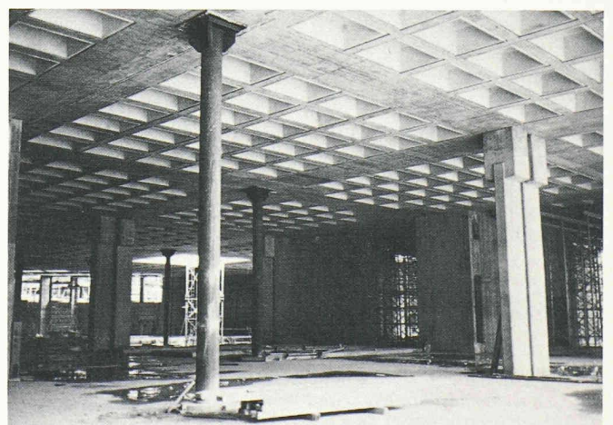
Fig. 14. — Colonne forgée avec chapiteau.
