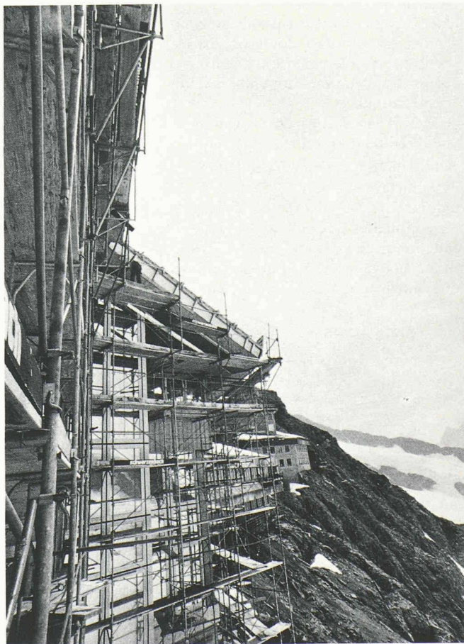
Fig. 9. — Vue prise durant le montage des façades. A la hauteur vertigineuse s'ajoute le vent soufflant bien plus fort qu'en plaine.
