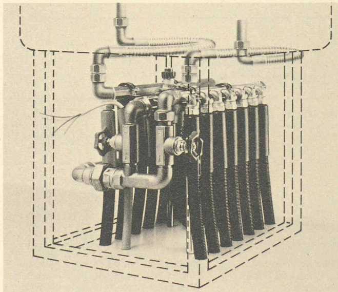
Fig. 4. - Exemple d'une installation posée terminée.
