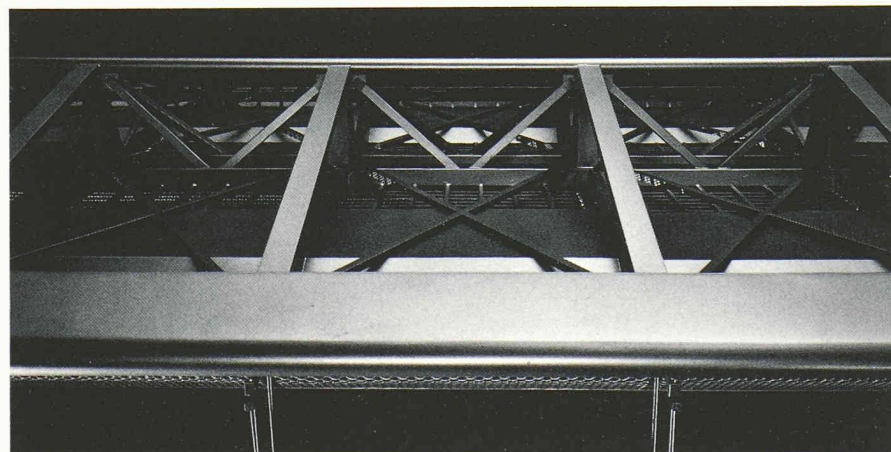
Fig. 5. — Détail de la construction du tablier du projet de la Société du détroit de Messine.
