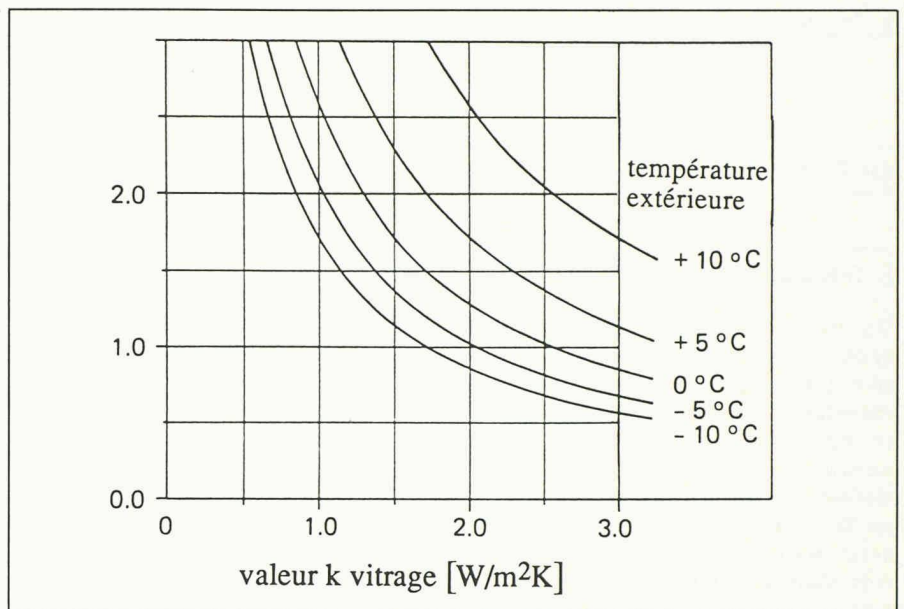
Fig. 2. — Hauteur maximale admissible d'une fenêtre sans radiateur sous la fenêtre ( V_{air, admissible} = 25 \text{ cm/s} ).
