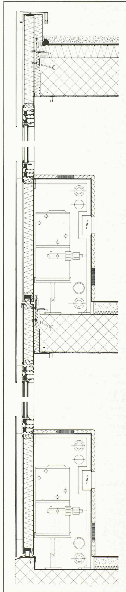
Coupe verticale.
