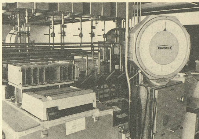
Interface balance-imprimante.
