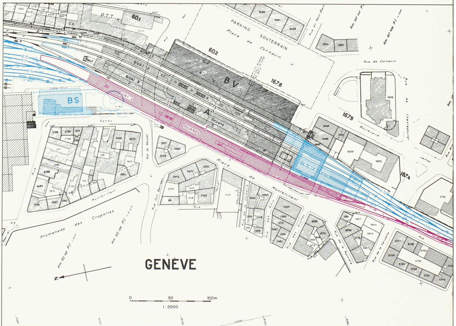
Fig. 1. - Plan de situation. En rouge, le quai 4 nouvellement créé.
