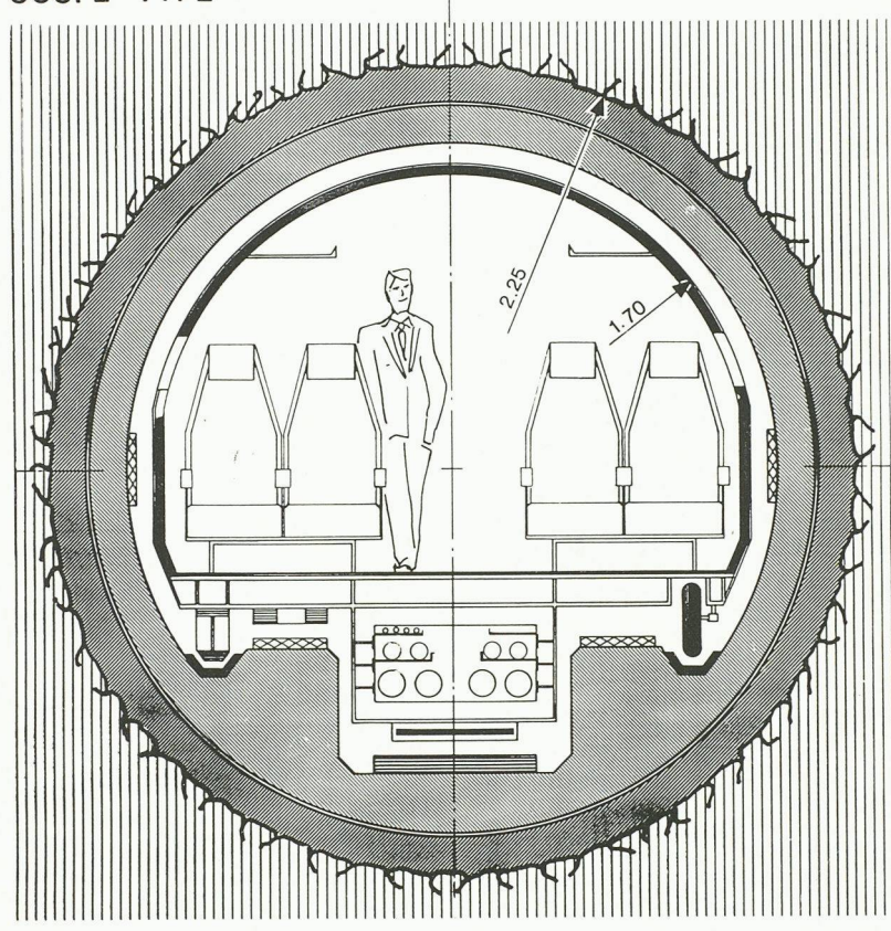
Fig. 1. — Coupe type du Swissmétró.
