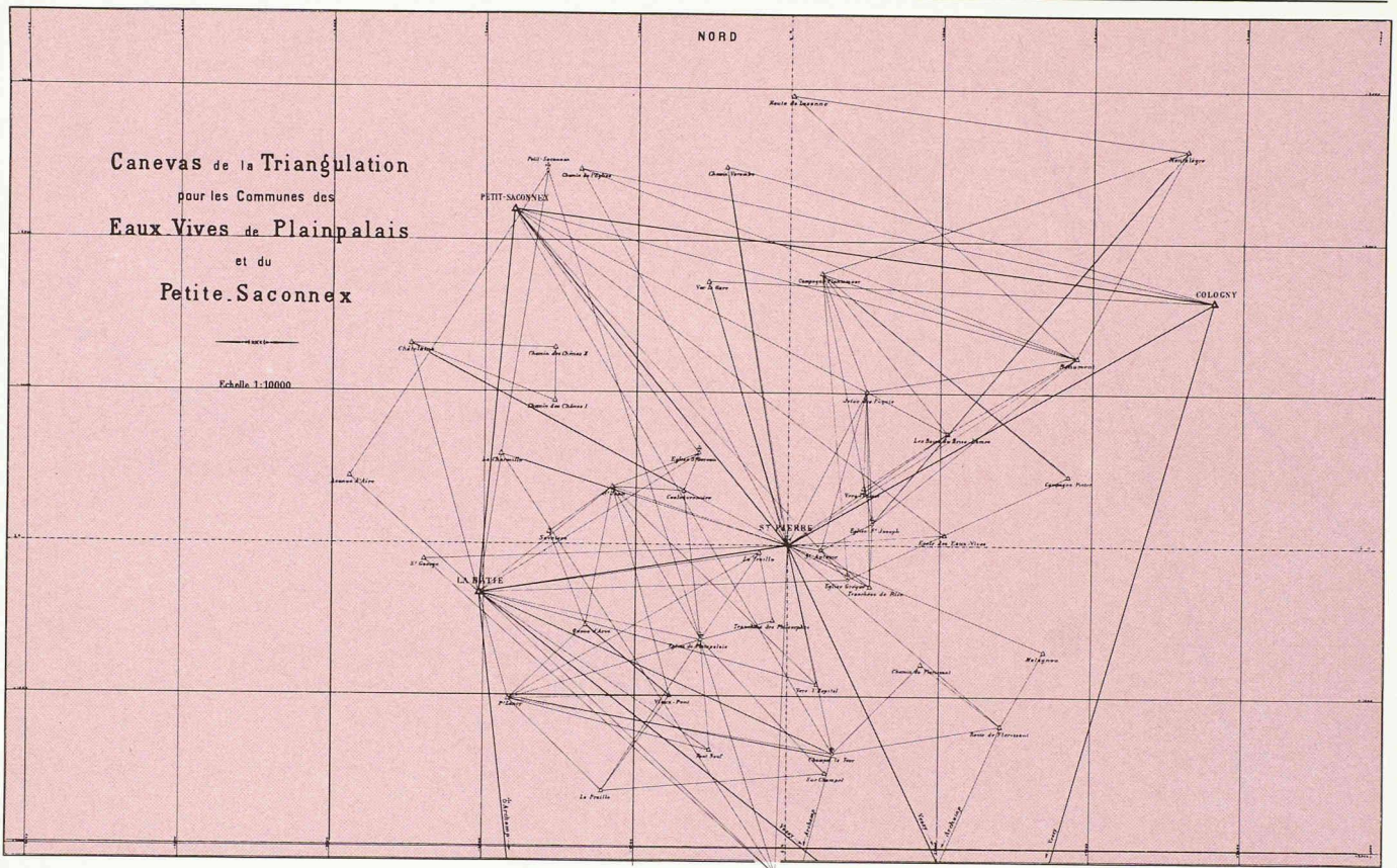
Fig. 6. – Canevas de la triangulation des communes genevoises, élaboré vers 1830 sous la direction de l'ingénieur cantonal Dufour. Le système de coordonnées géodésiques part alors de la tour nord de la cathédrale Saint-Pierre. Les repères géodésiques étaient exposés aux dégradations commises par des citoyens ignares. «[...] la triangulation de 1838-1841 avait dû être refaite spécialement, parce qu'il n'était rien ou presque rien resté des anciens repérages des points trigonométriques. Nous trouvons bien aujourd'hui dans les archives des calculs exacts, méticuleusement opérés, et des valeurs de coordonnées qui correspondraient encore aujourd'hui aux exigences les plus sévères; mais que sont devenus les repérages des points? On n'en trouve plus trace!» (H. Zoelly vers 1910.)
