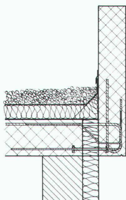
ISOKORB type F
