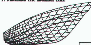
EXEMPLE D'IMPORTATION DE FICHIERS DXF (AUTOSHIP) ET D'IMPRESSION AVEC IMPRIMANTE LASER
