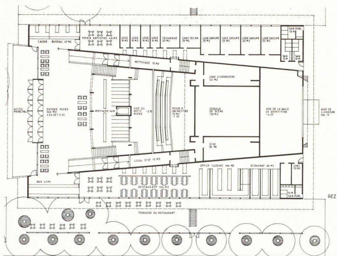
Rez-de-chaussée 1:750
