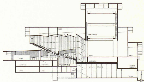
Coupe longitudinale
