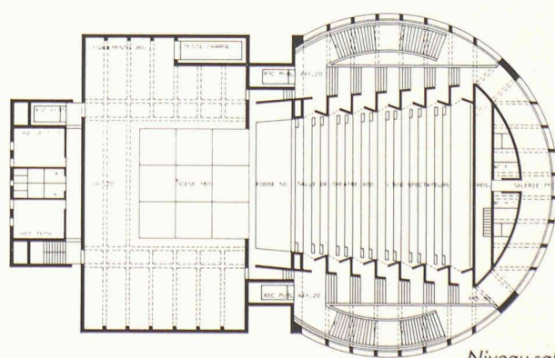
Niveau salle
