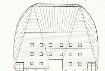
Façade est
