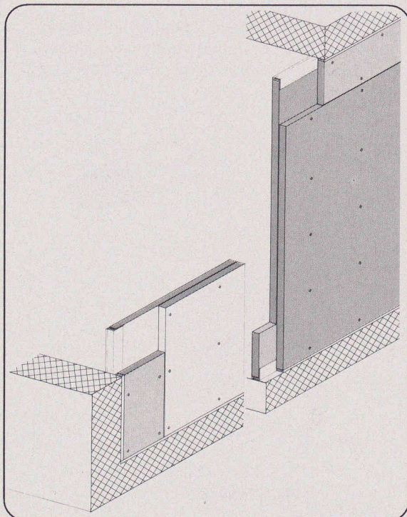
Parois de séparation PROMATECT-H, e = 2 \times 20 \text{ mm}
