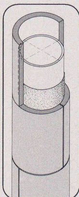
Revêtement de piliers circulaires PROMASIL, e = 40 \text{ mm}
