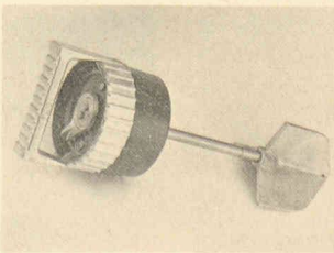
Plasticimètre P 86.
