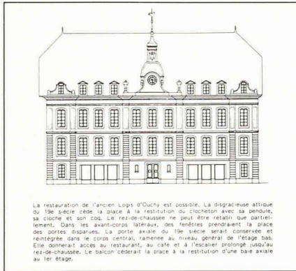
Fig. 54 et 55. Le Logis d'Ouchy (Hôtel d'Angleterre), 1775-1779, par l'architecte Abraham Fraisse. Elevation de la façade sud, restituée, et plan du second étage, état actuel. Echelle 1:200.
