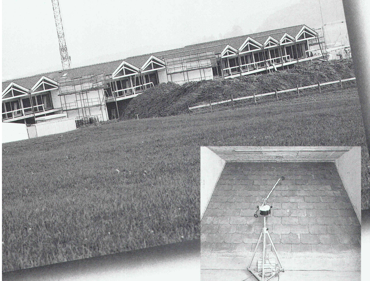
Test d'impact aux bruits aériens sur modèle réel. EMPA Zurich.
