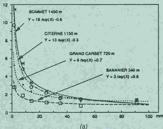
Figure 7 : (a) Courbes d'ajustement de la décroissance de l'accroissement orographique en fonction de la précipitation à Capesterre. (b) Effet orographique en fonction de l'altitude et de la pluviométrie à Capesterre.
