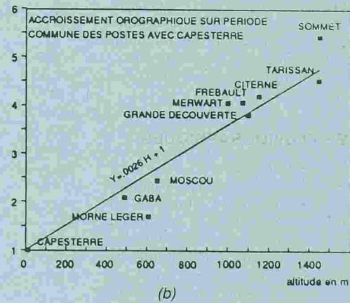
Figure 5: (a) Influence orographique moyenne (période commune pour tous les postes). (b) Vérification sur d'autres postes (périodes communes avec Capesterre deux à deux)
