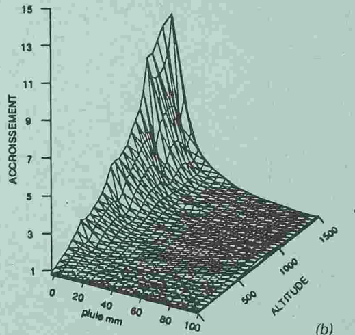
Figure 7 : (a) Courbes d'ajustement de la décroissance de l'accroissement orographique en fonction de la précipitation à Capesterre. (b) Effet orographique en fonction de l'altitude et de la pluviométrie à Capesterre.
