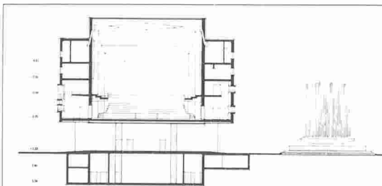
Coupe de la salle
