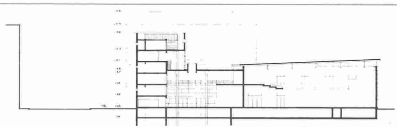
Coupe du foyer
