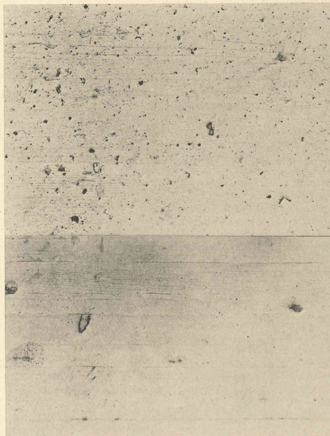
En haut: surface de béton dont le coffrage n'a pas été préparé. De grosses inclusions d'air sont visibles. En bas: coffrage traité avec Rheofinish; il en résulte une surface de béton sans pores.
