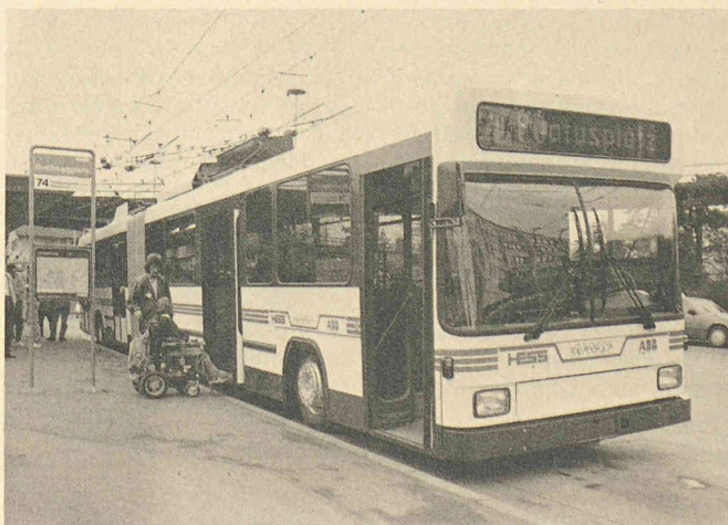
Le «Swisstrolley», le premier trolleybus articulé du monde doté d'un plancher surbaissé, facilite aux personnes âgées, se déplaçant avec difficulté ou en chaise roulante, ainsi qu'aux personnes accompagnées d'un enfant dans un landau, l'accès au véhicule.
