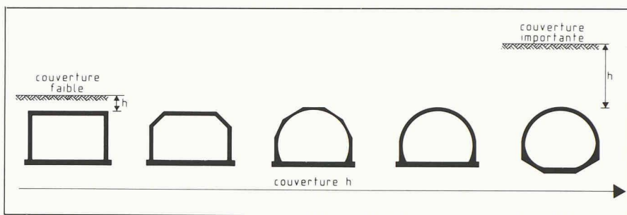
Fig. 4. - Galeries couvertes : adaptation de la section transversale à la couverture de terrain.
