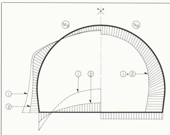
Fig. 5. - Galerie couverte, influence d'une adaptation des rigidités. El. ① rigidité E_c I_c ; ② rigidité adaptée.
