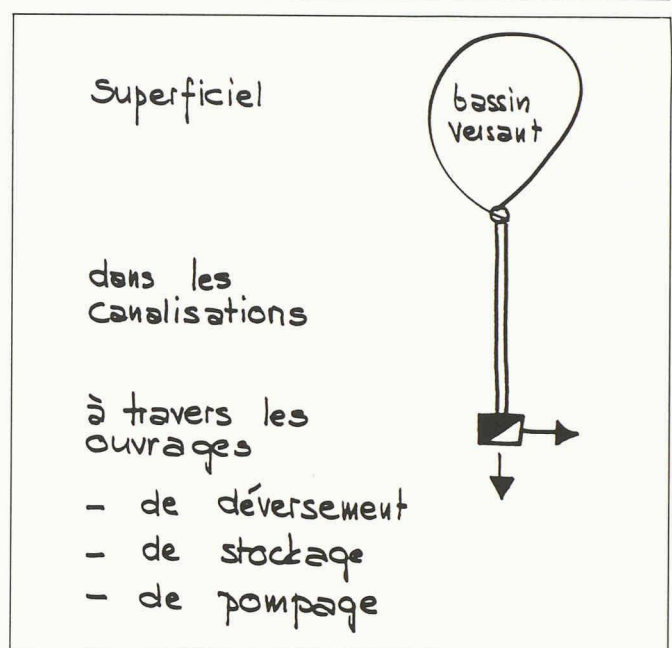
Fig. 9. - Modèles d'écoulement.
