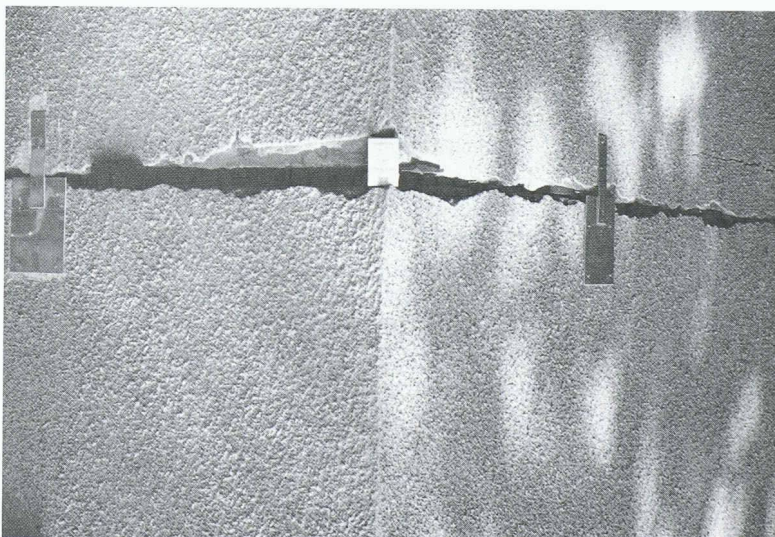
Fig. 4. – Détail de la fissure à l'angle du bâtiment
